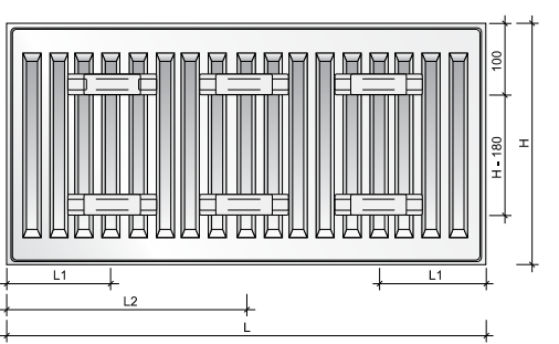
Вид сзади
