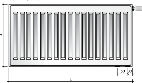
Вид спереди
